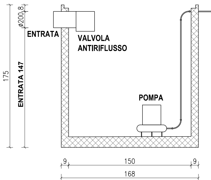
SEZIONE AA
