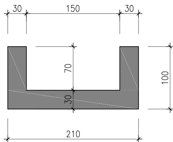
SEZIONE A-A
